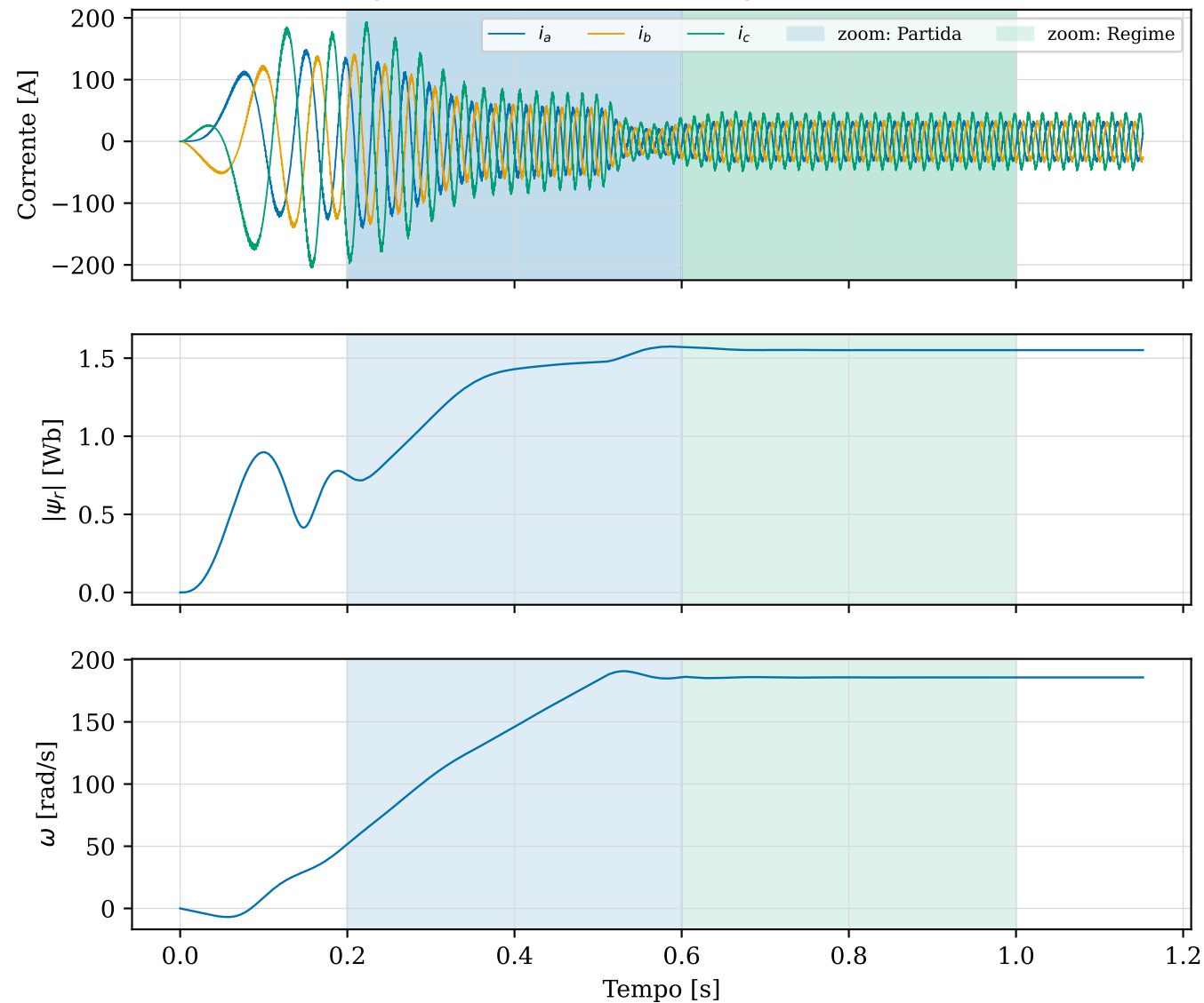
L4 — B2 — degrau 0,50→1,00 T_n : visão geral da captura (FPGA real)
