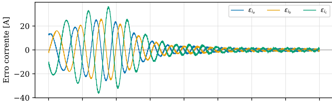
L4 — B2 — degrau 0,50→1,00 T_n · Partida: erro FPGA (real) — Modelo C
