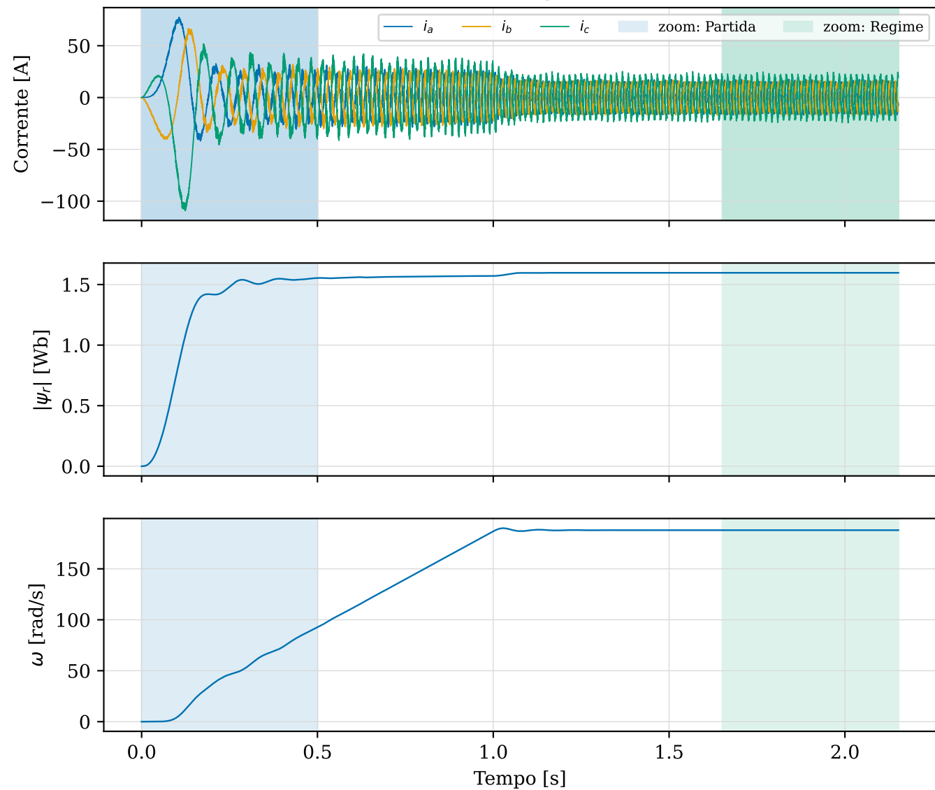
L4 — S0 — t_{acc}=1 s, vazio: visão geral da captura (FPGA real)
