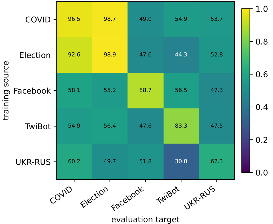
MT ROC-AUC (%)
