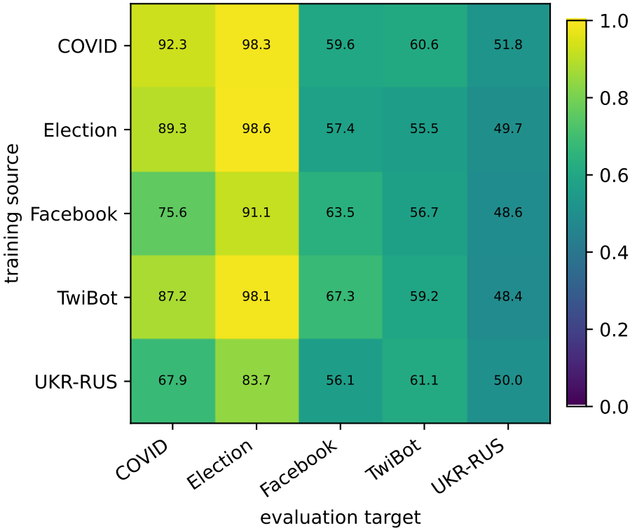
NM ROC-AUC (%)
