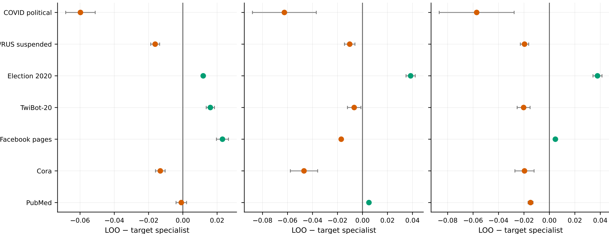
Macro OVR AUC
