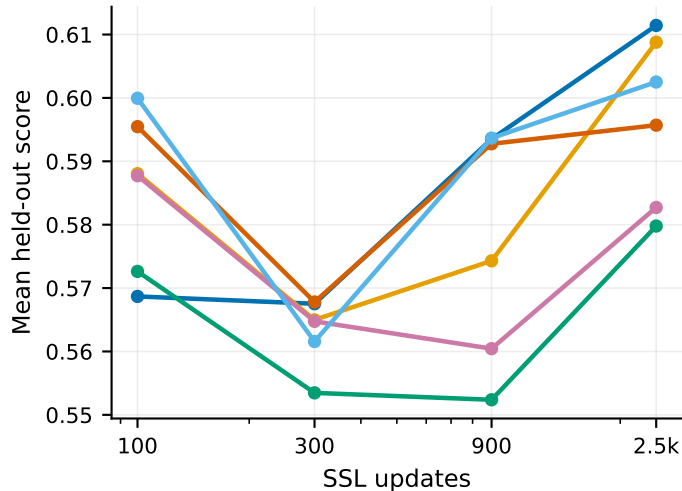
Macro F1
