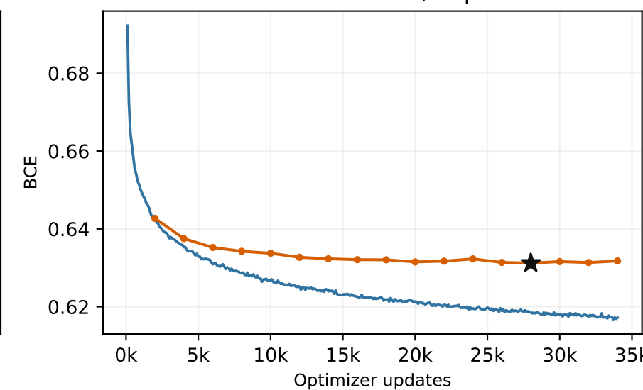
Facebook · best 28k / stop 34k
