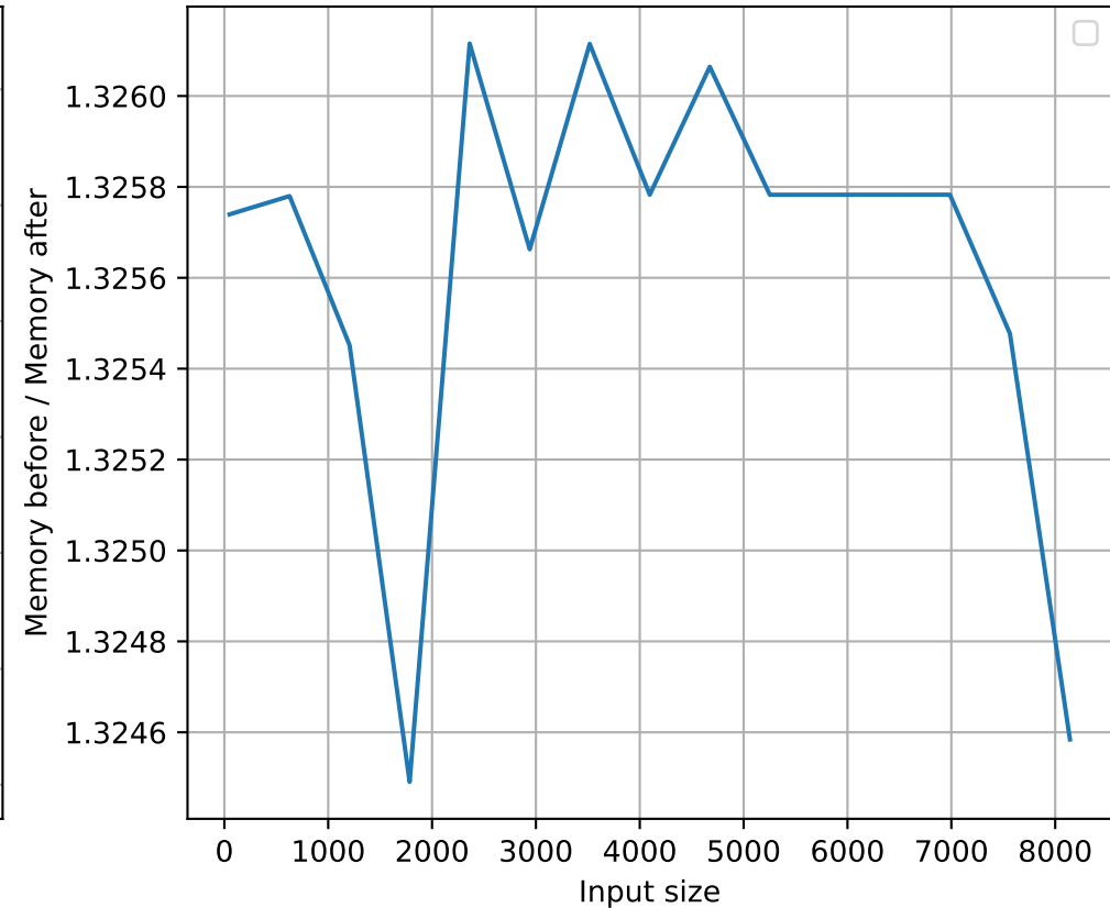
Mistral-7B-v0.1
