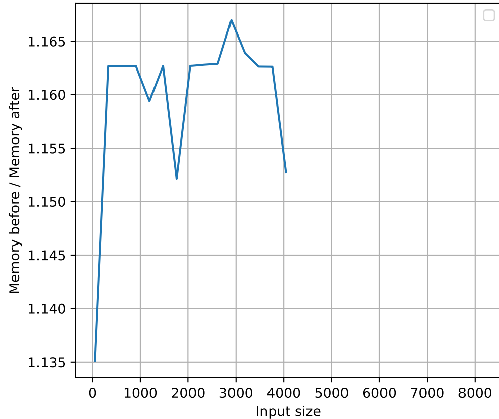
Llama-2-7b-hf
