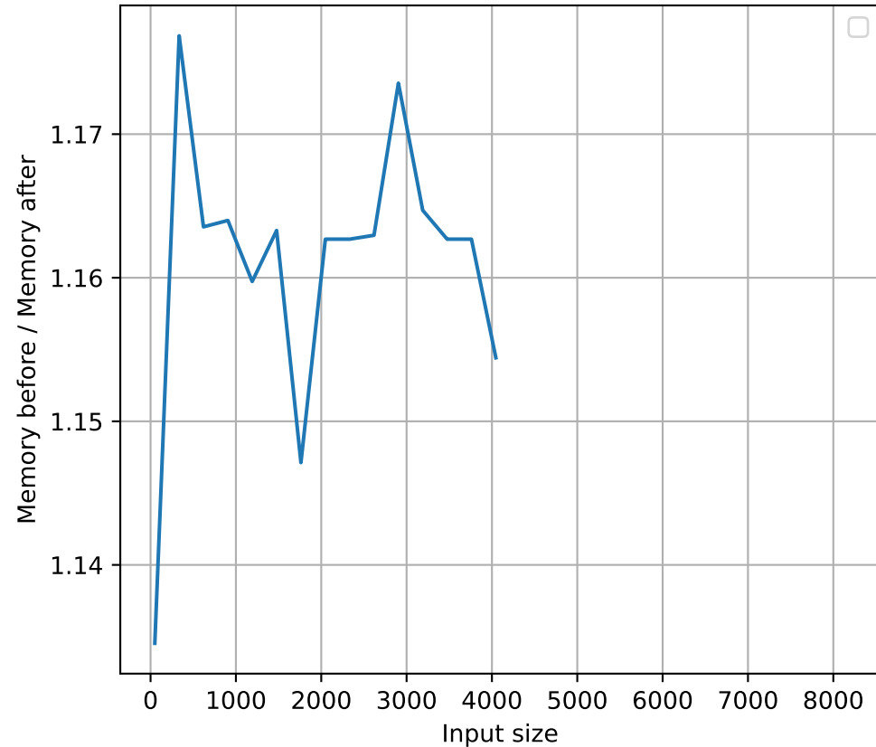
Llama-2-7b-hf
