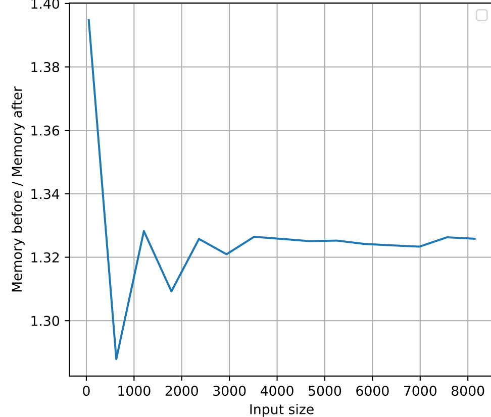
Mistral-7B-v0.1
