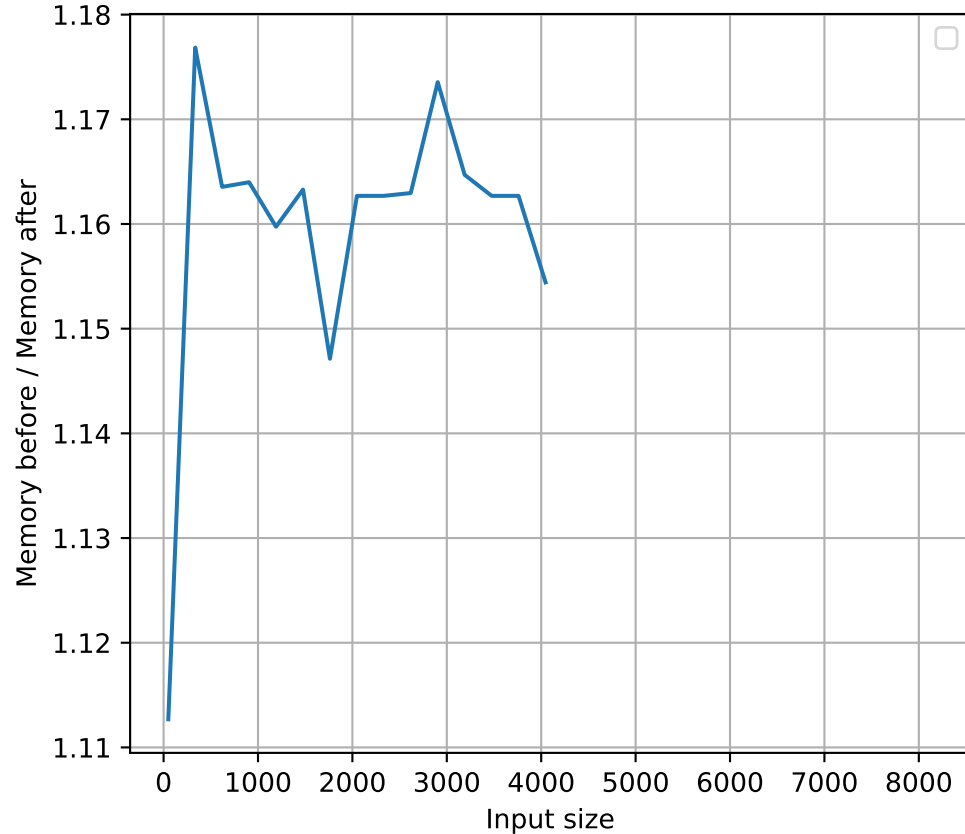
Llama-2-7b-hf
