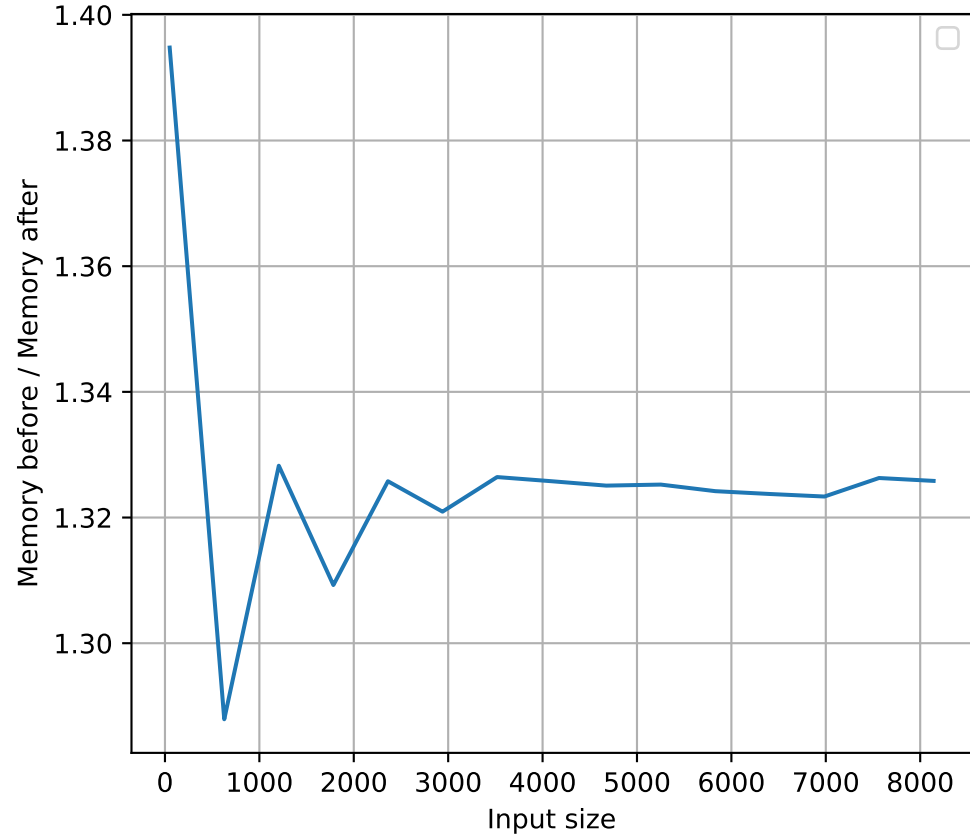
Mistral-7B-v0.1
