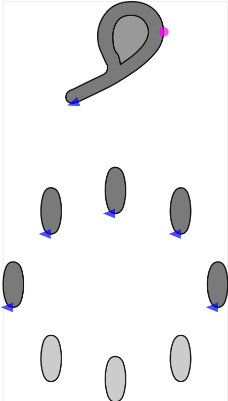
'wght=200.0'
