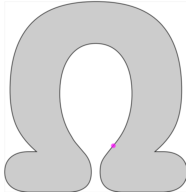
'wght=900.0'
