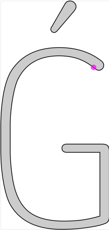
'wght=200.0'
