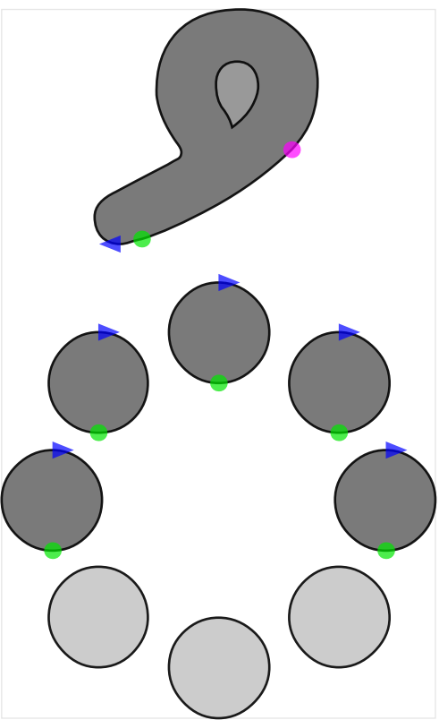
'wght=900.0'
