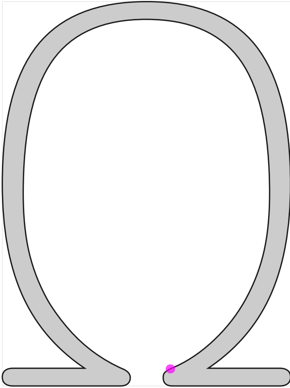
'wght=200.0'
