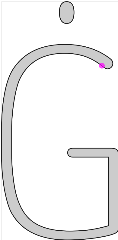
'wght=200.0'
