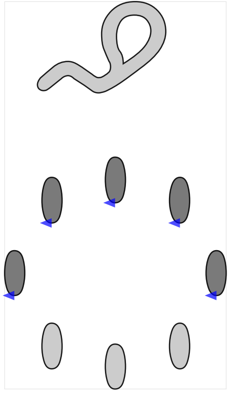
'wght=900.0'
