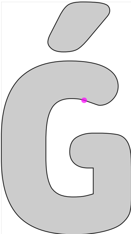
'wght=900.0'
