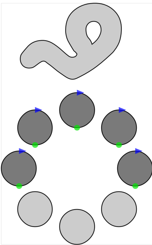
'wght=900.0'
