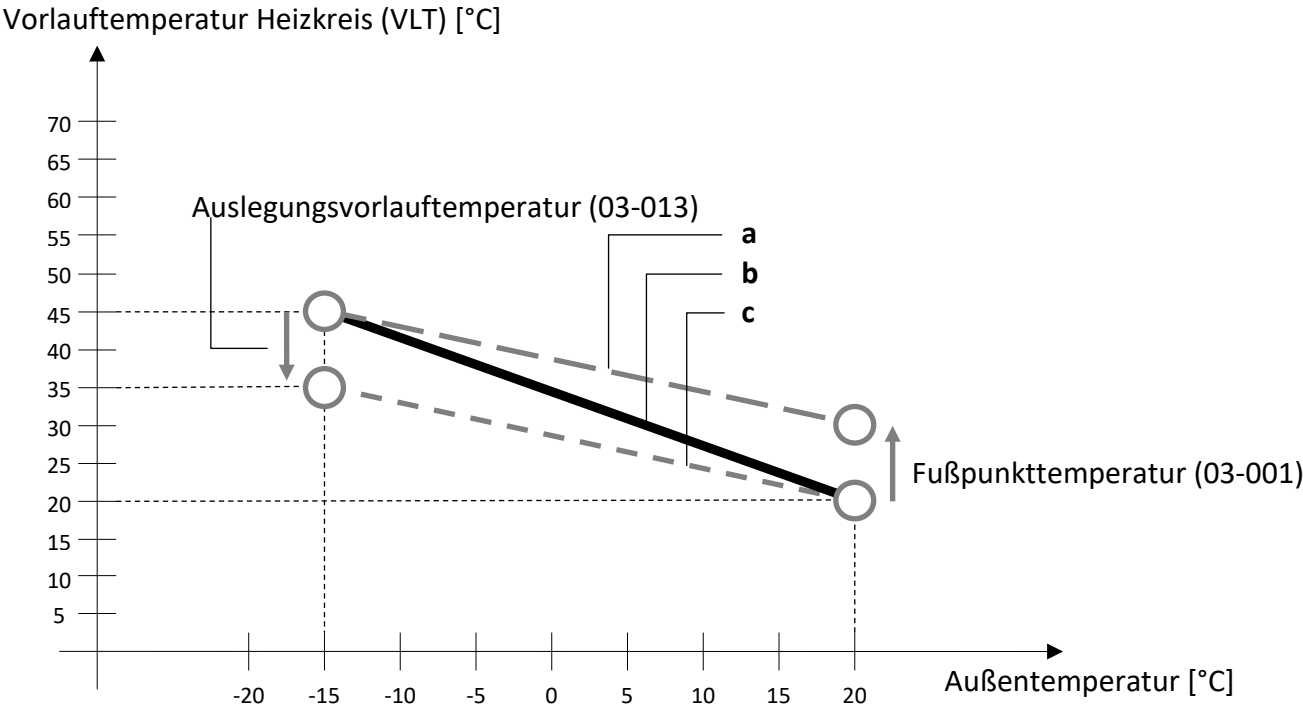
Abbildung 9: Heizkurve Korrektur
