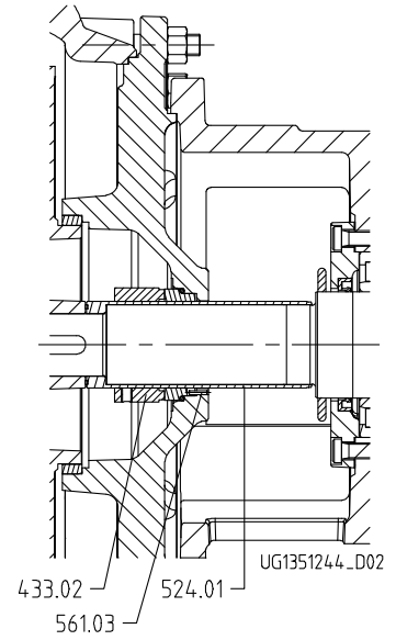
Cierre mecánico con tapa de carcasa cónica
