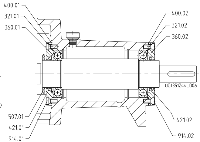
Ejecución con lubricación con aceite (cojinetes económicos)
