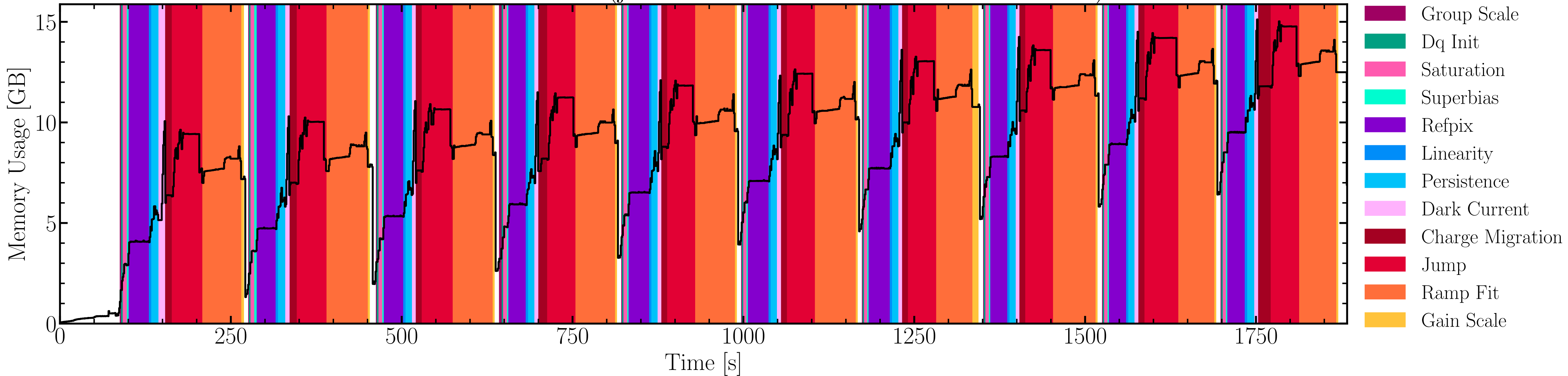
NIRISS-WFSS: 125.9 MB (jw04681446001_06201_00002_nis_uncal.fits)
