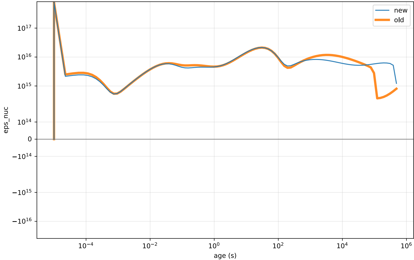
approx21_plus_co56 zspllit_3GK
