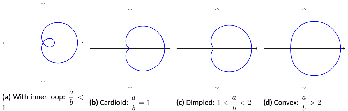
Figure 10.4.20 Limaçons
