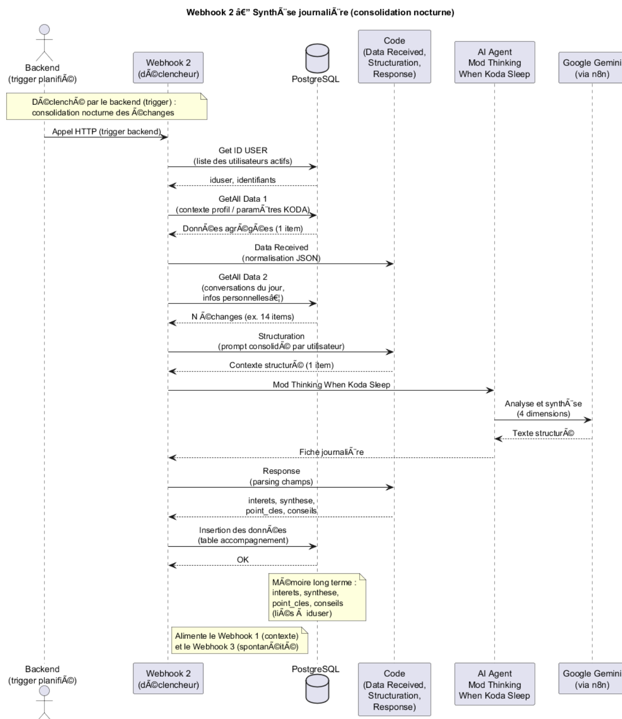
FIGURE III.30 – Webhook 2 — diagramme de sâ€¢quence (synthâ€¢se journaliâ€¢re et persistance)
