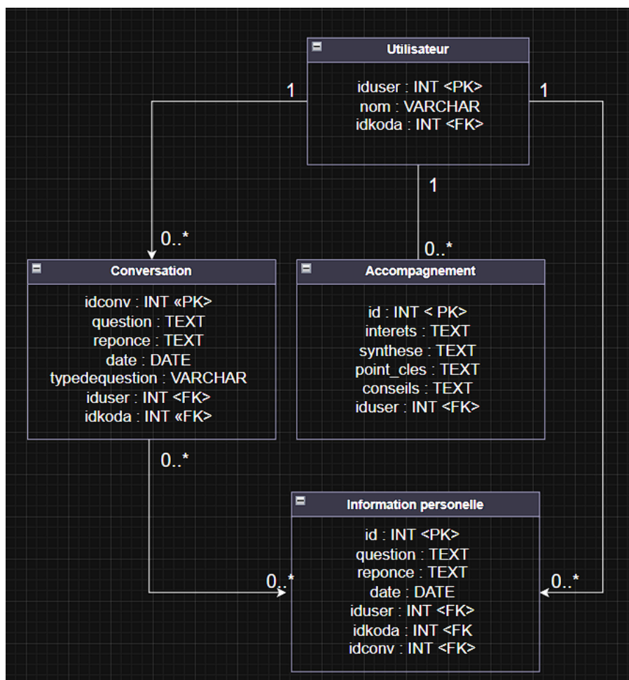
FIGURE III.32 – Webhook 2 — schéma de persistance (utilisateur → accompagnement : interets, synthese, point_cles, conseils)
