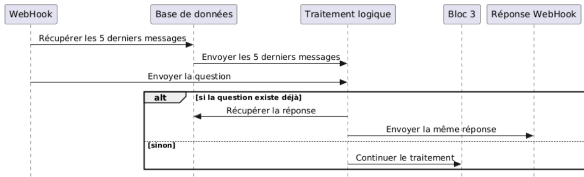
FIGURE III.10 – Block 2 — Diagramme de séquence du deuxième bloc
