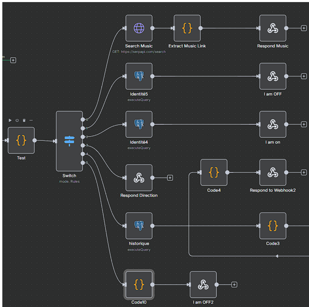
FIGURE III.6 – Block 1 — Workflow n8n : nœud Code Test , Switch à six sorties (musique SerpAPI, identité ON/OFF, direction, historique, branche dédiée)
