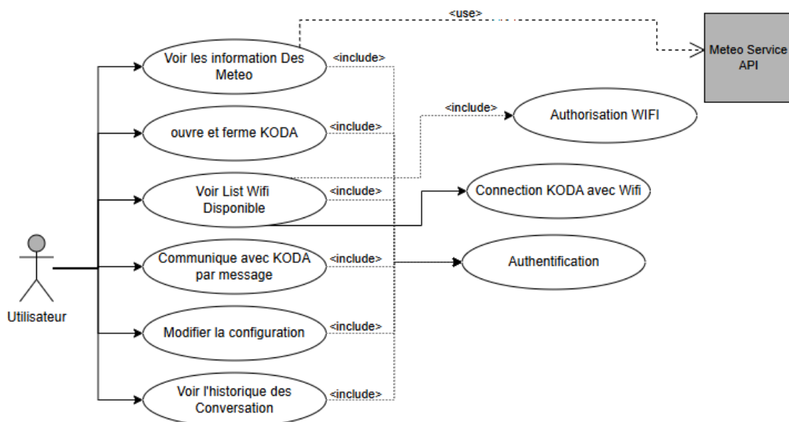
FIGURE VII.1 – KodaMate — diagramme de cas d'utilisation global (chapitre VII)
