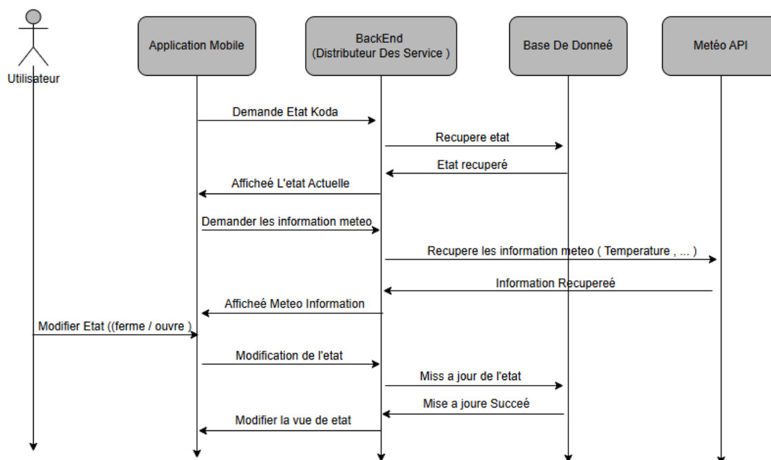
FIGURE VII.7 – KodaMate — séquence écran d'accueil (dshome)
