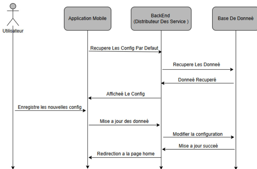
FIGURE VII.5 – KodaMate — séquence configuration initiale après login (dsconfiglogin)
