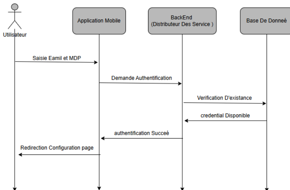
FIGURE VII.3 – KodaMate — séquence de connexion (dslogin)
