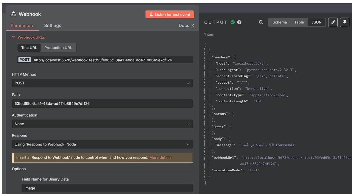
FIGURE IV.15 – Communication avec n8n — exemple de payload en entrée de webhook (Webhook 1)
