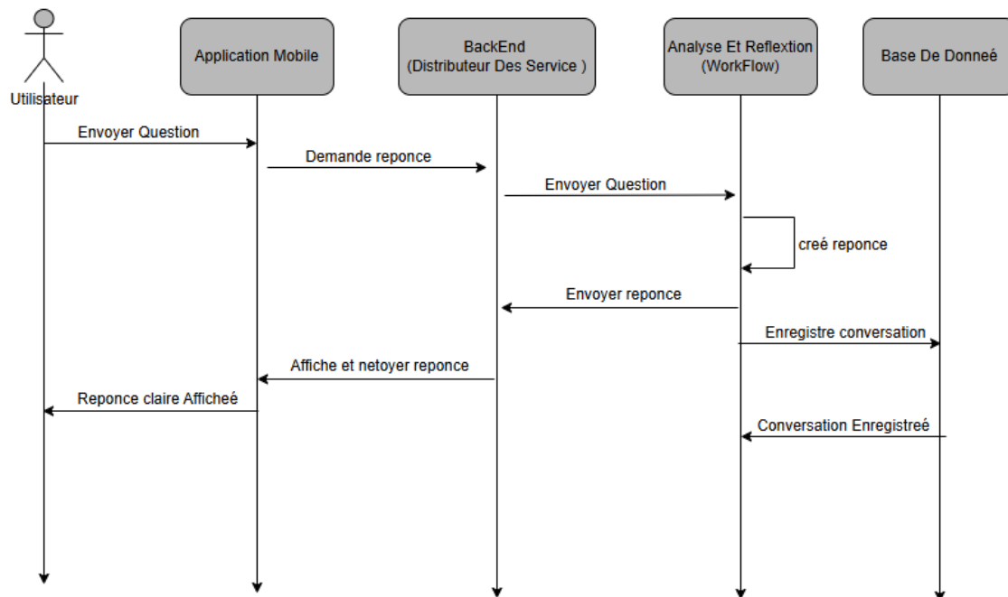
FIGURE VII.9 – KodaMate — séquence écran de chat (dschat)
