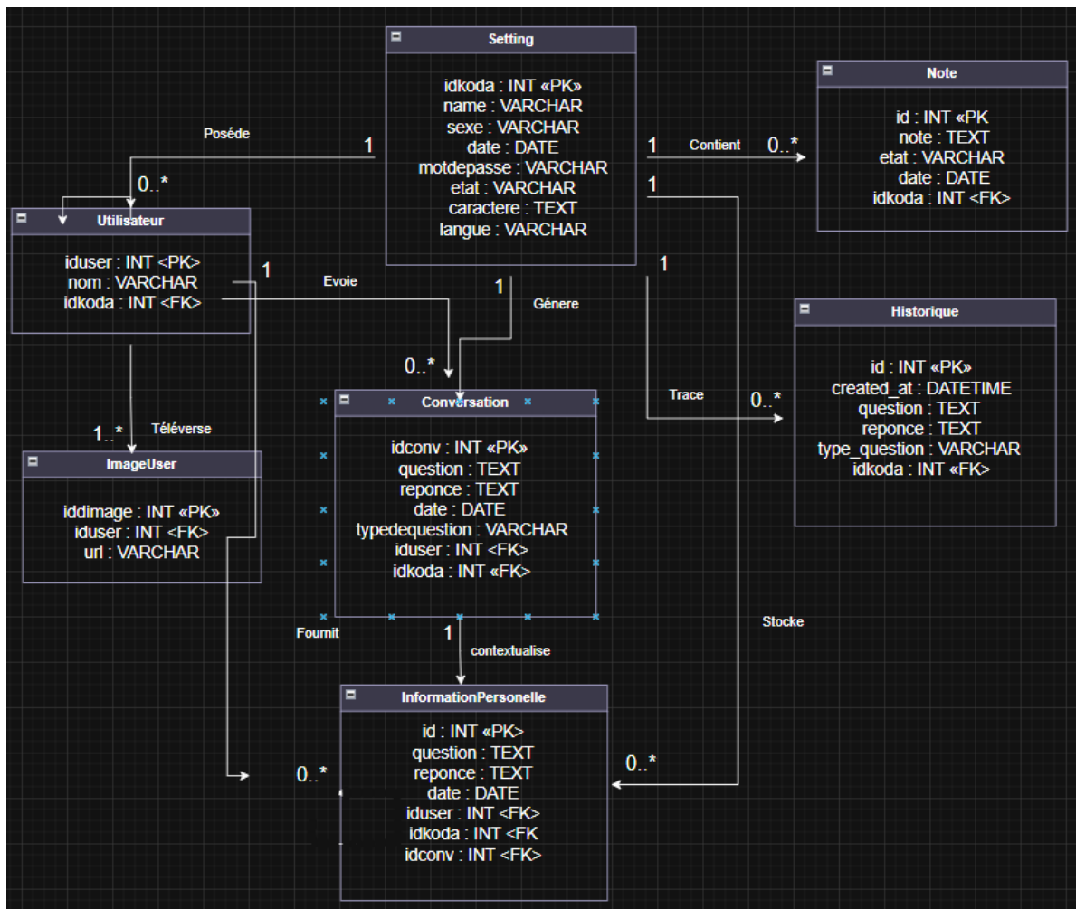
FIGURE IV.2 – Cycle 2 — schéma de classes et modèle de persistance (PostgreSQL)
