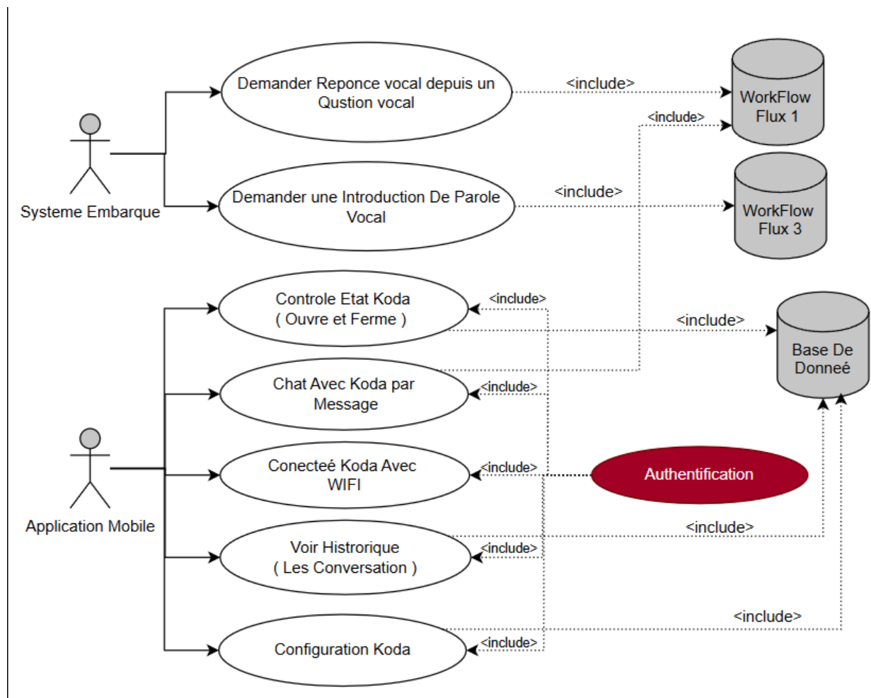
FIGURE IV.1 – Cycle 2 — diagramme de cas d'utilisation général du Distributeur de services
