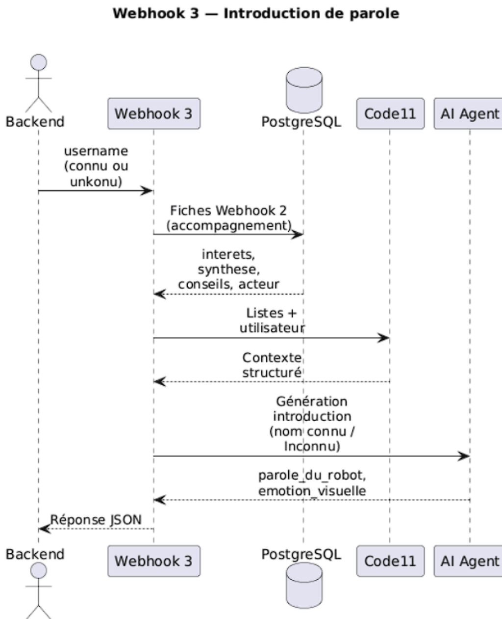
FIGURE IV.17 – Webhook 3 — diagramme de séquence (rappel)
