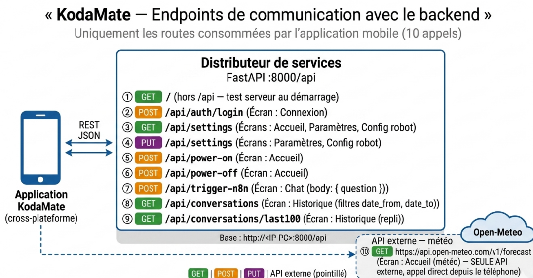
FIGURE IV.11 – Routes REST du Distributeur (vue globale)
