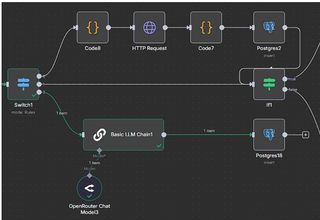
FIGURE III.19 – Gestion utilisateur (unkonu) — Switch1 , branche enregistrement (presentation), branche LLM (unkonu) et poursuite vers la réponse contextualisée
