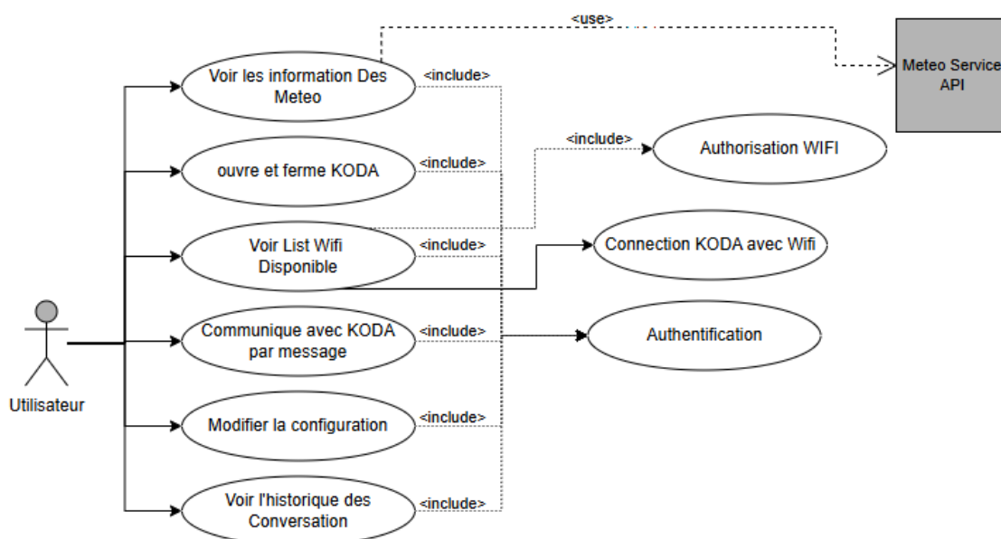
FIGURE VII.1 – KodaMate — diagramme de cas d'utilisation global (chapitre VII)
