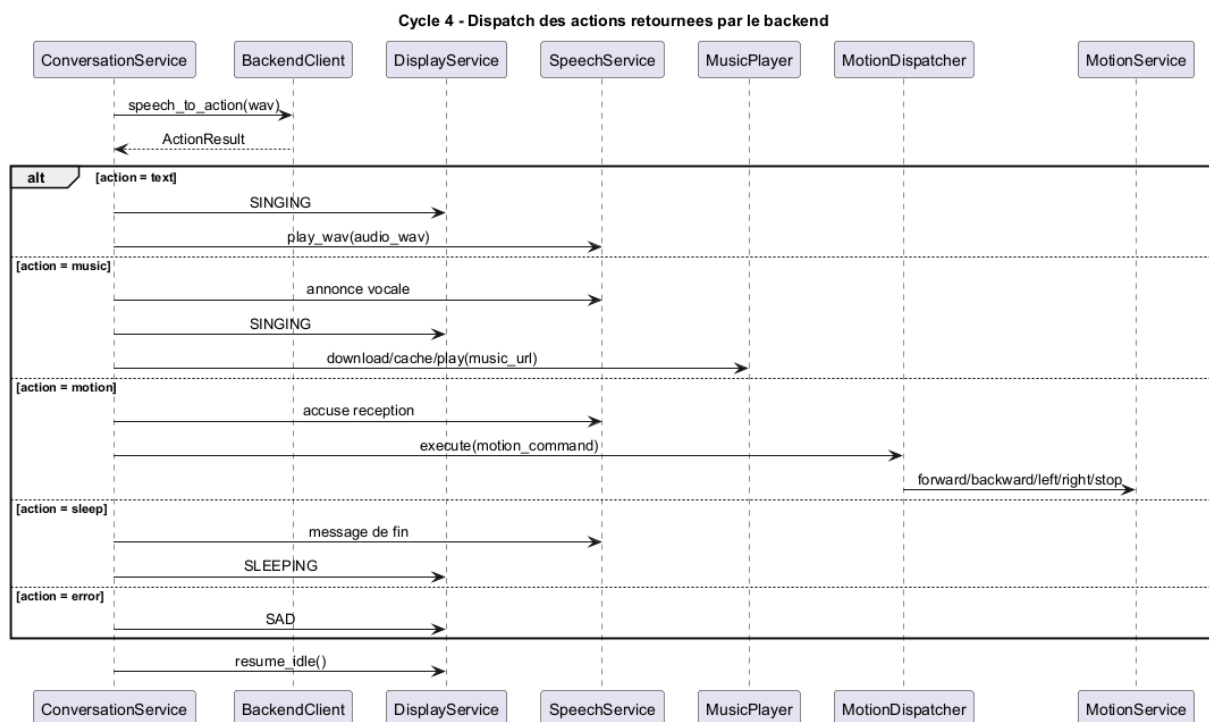
FIGURE VI.10 – Cycle 4 — dispatch des actions retournees par le backend
