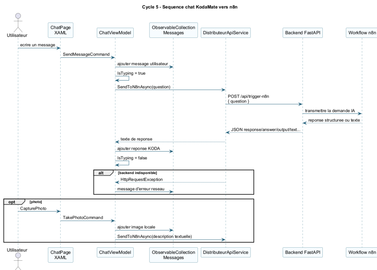
FIGURE VII.8 – Cycle 5 — séquence chat KodaMate vers n8n
