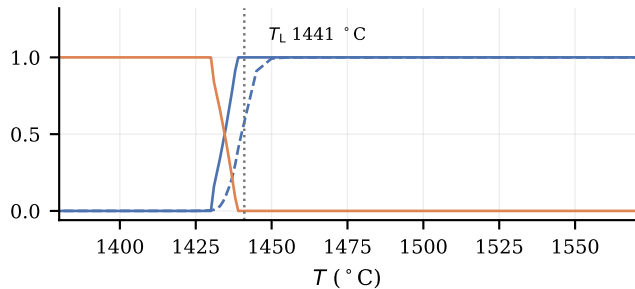
(d) Yamada Y: Cr 21, Ni 16.6 (bal. Fe)
