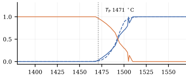
(d) Yamada Y: Cr 21, Ni 16.6 (bal. Fe)
