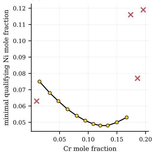
(b) Pareto frontier: Ni minimum vs Cr
