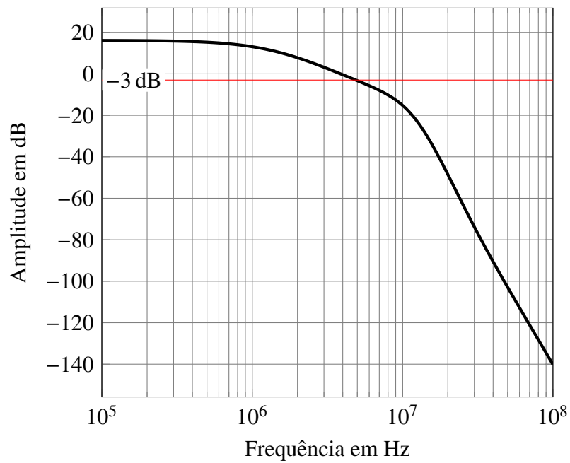
Figura 3.2: Análise AC da saída do estágio de ganho.
