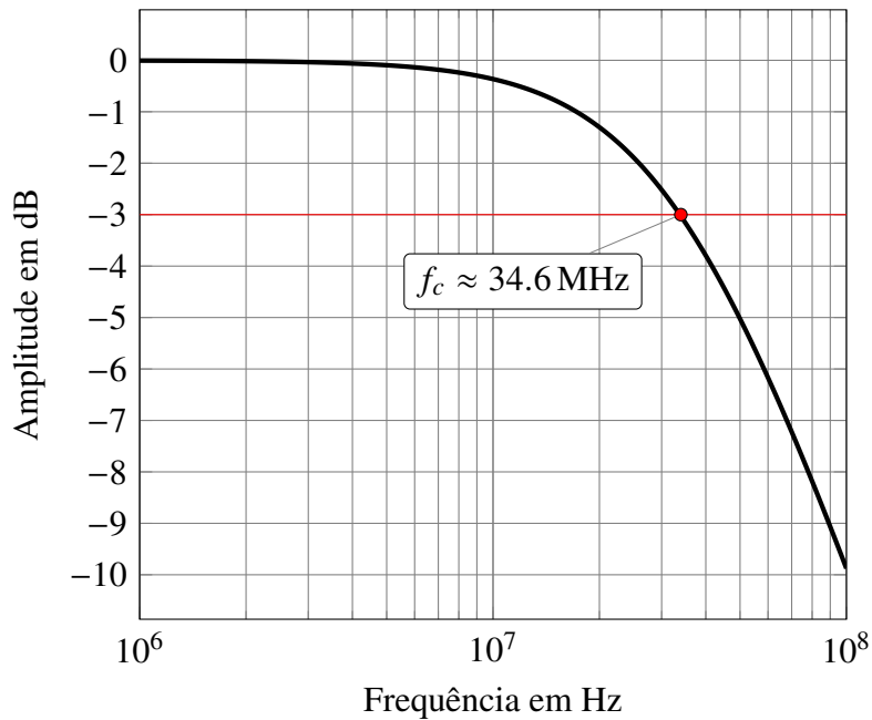
Figura 3.1: Análise AC da saída da entrada desbalanceada.
