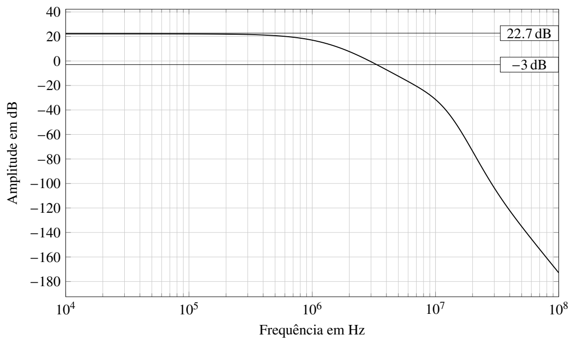
Figura 2.2: Análise AC da saída do estágio de ganho.
