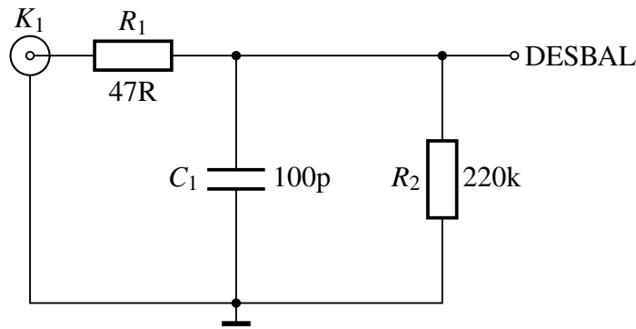
Figura 1.1: Esquemático da entrada desbalanceada.
