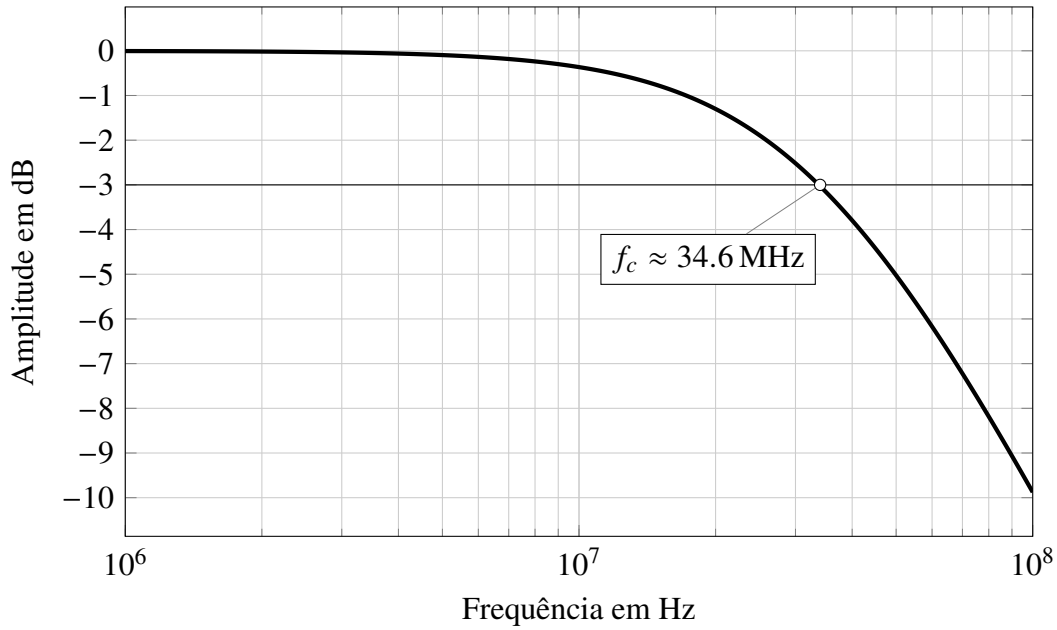
Figura 2.1: Análise AC da saída da entrada desbalanceada.
