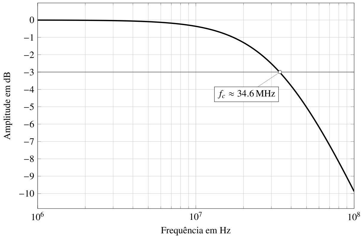
Figura 3.1: Análise AC da saída da entrada desbalanceada.
