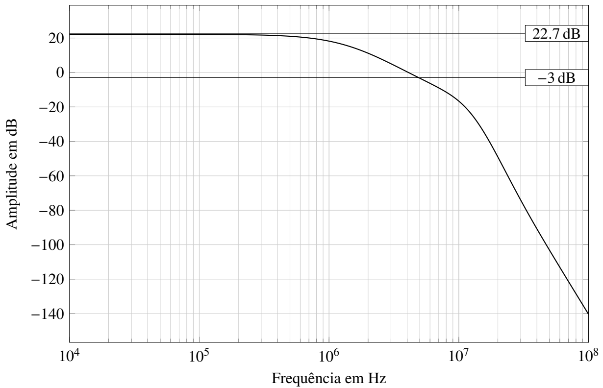
Figura 3.2: Análise AC da saída do estágio de ganho.
