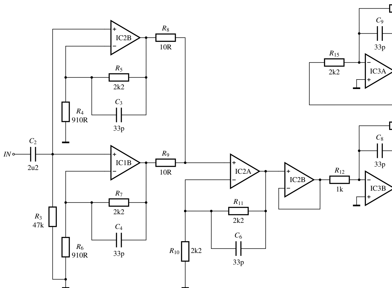
Figura 3.4: Esquemático do estágio de ganho.
