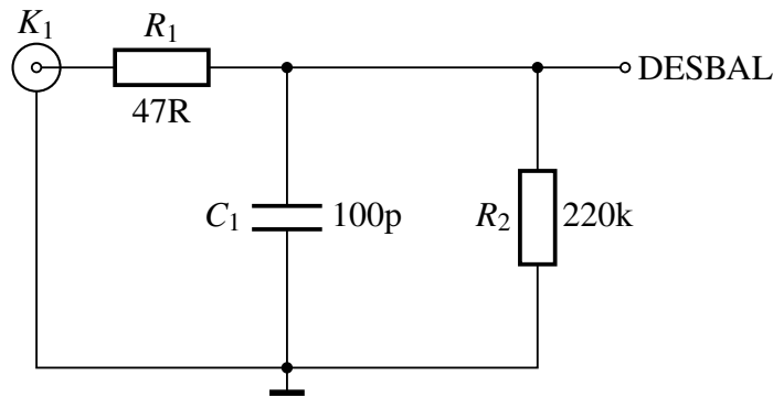
Figura 1.1: Esquemático da entrada desbalanceada.
