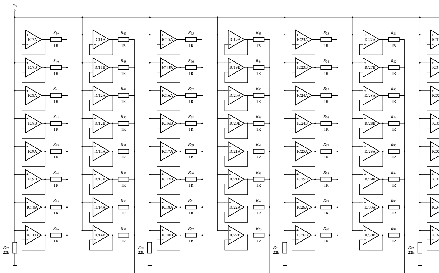
Figura 3.5: Estágio de potência.
