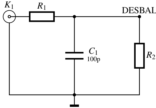
Figura 3.1: Esquemático da entrada desbalanceada.
