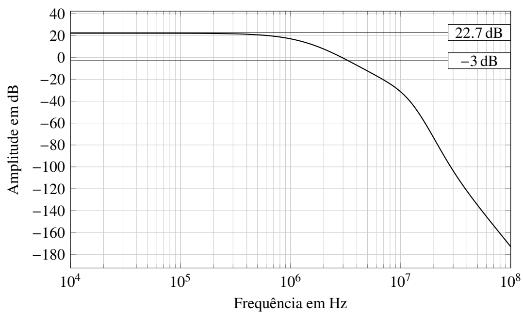
Figura 3.4: Análise AC da saída do estágio de ganho.
