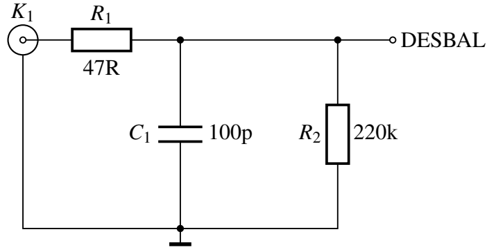
Figura 2.1: Esquemático da entrada desbalanceada.
