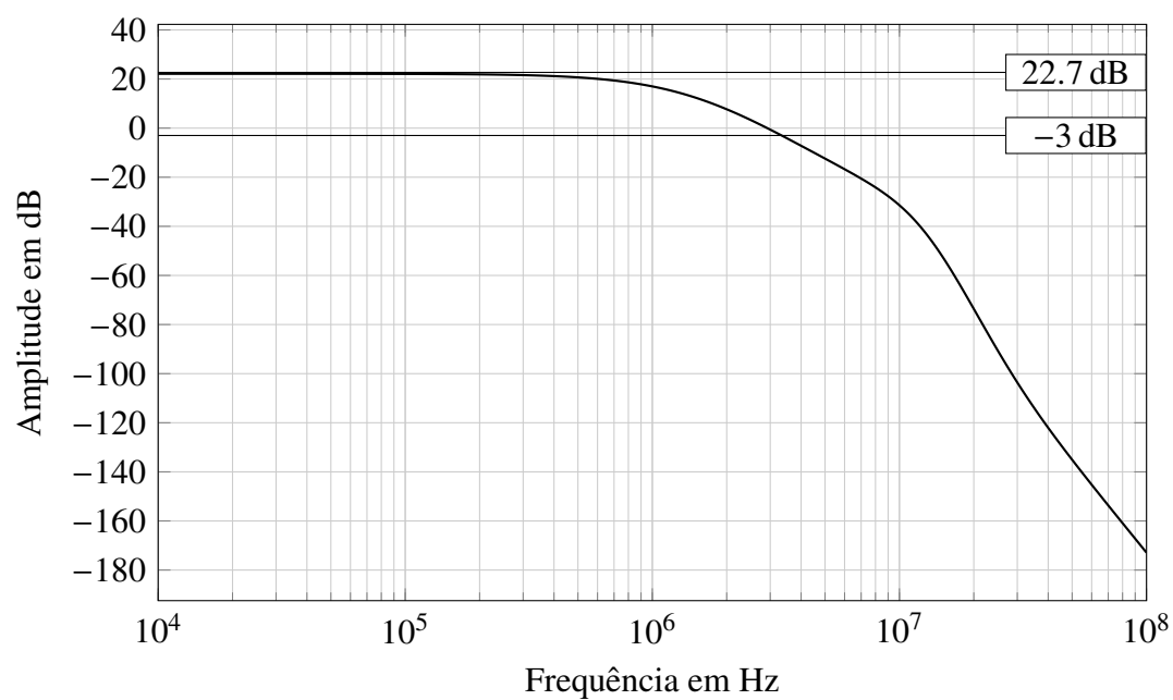
Figura 3.2: Análise AC da saída do estágio de ganho.
