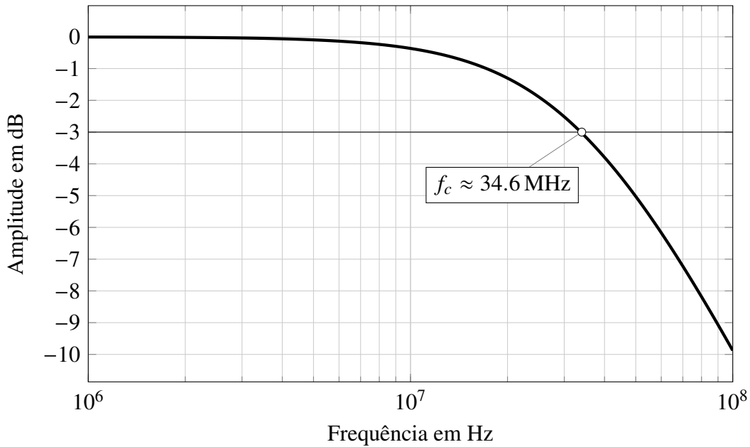
Figura 3.1: Análise AC da saída da entrada desbalanceada.
