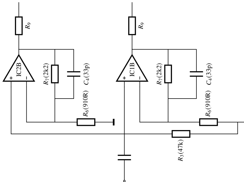
Figura 3.3: Esquemático da entrada desbalanceada
