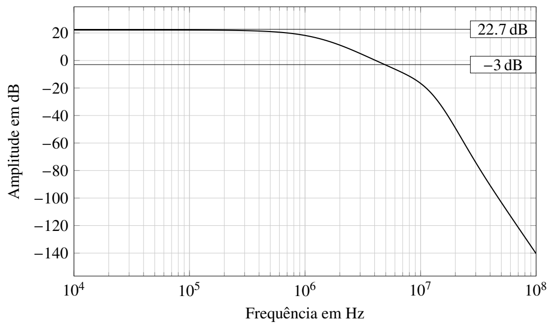
Figura 3.2: Análise AC da saída do estágio de ganho.
