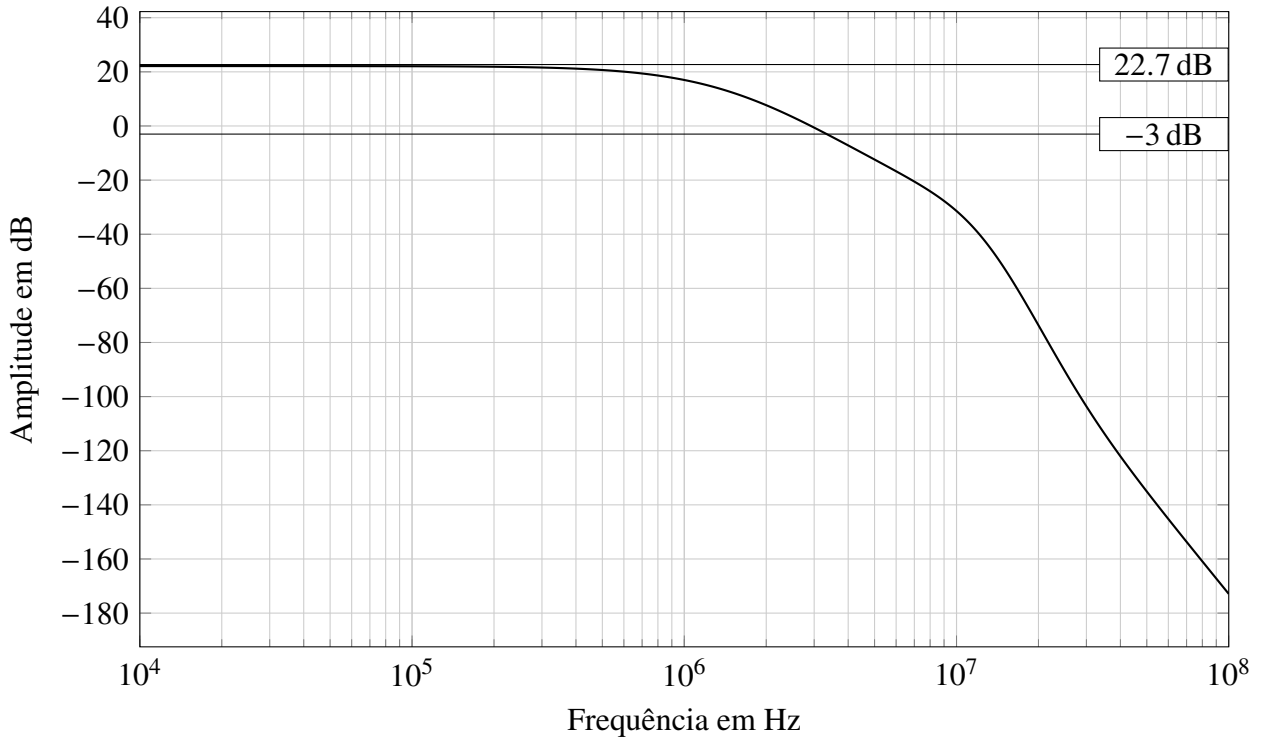
Figura 2.3: Análise AC da saída do estágio de ganho.
