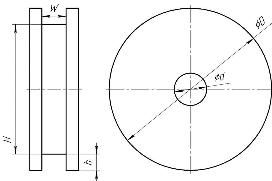
Рисунок 2.1 — Модель шкива с размерами
