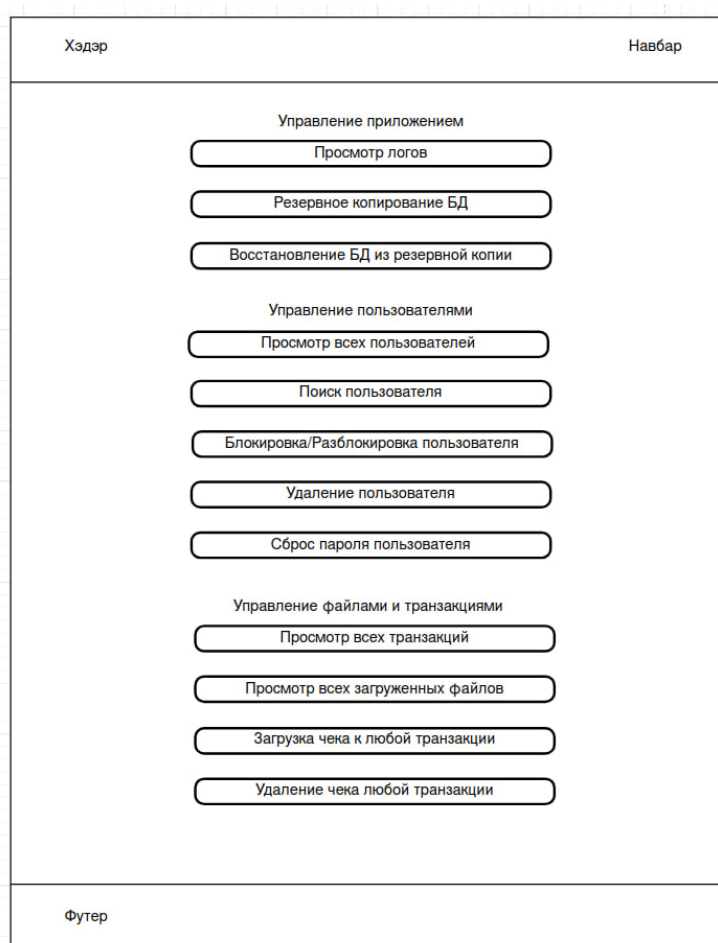
Рисунок 2.10 – Макет дашборда для администратора
