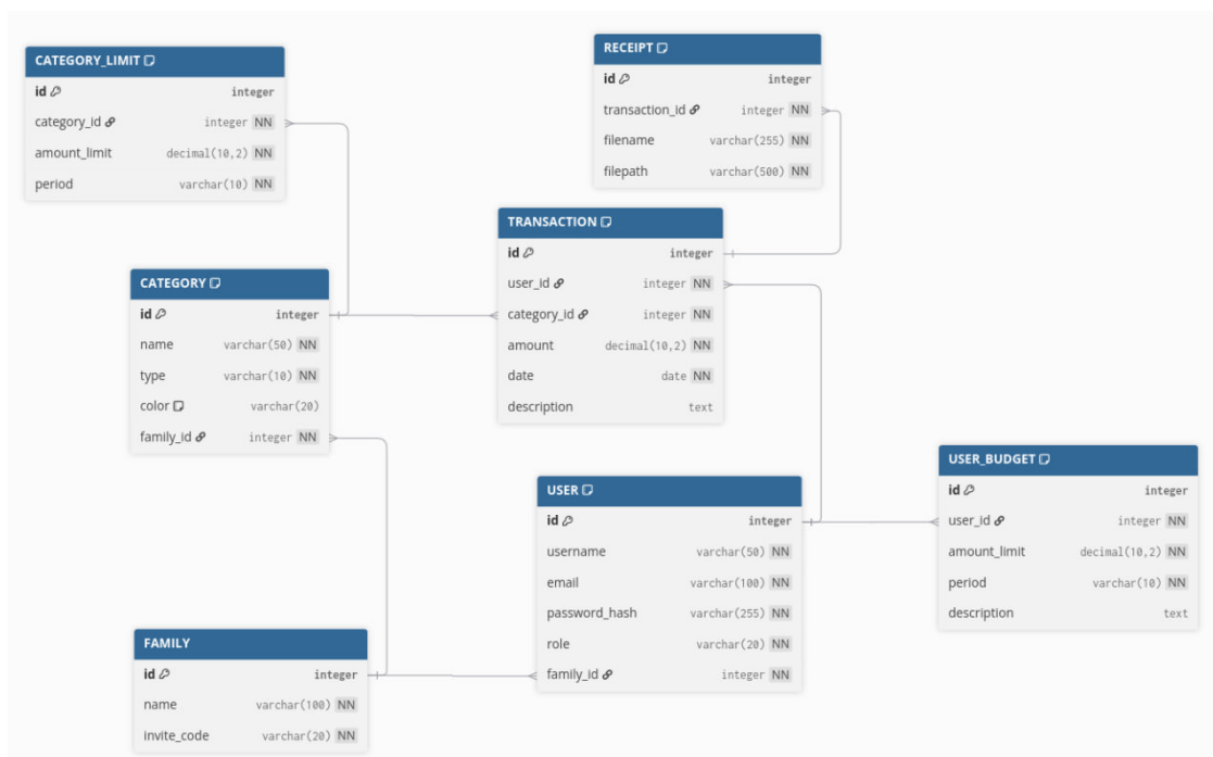
Рисунок 2.7 – ER-диаграмма базы данных веб-приложения для ведения семейного бюджета
