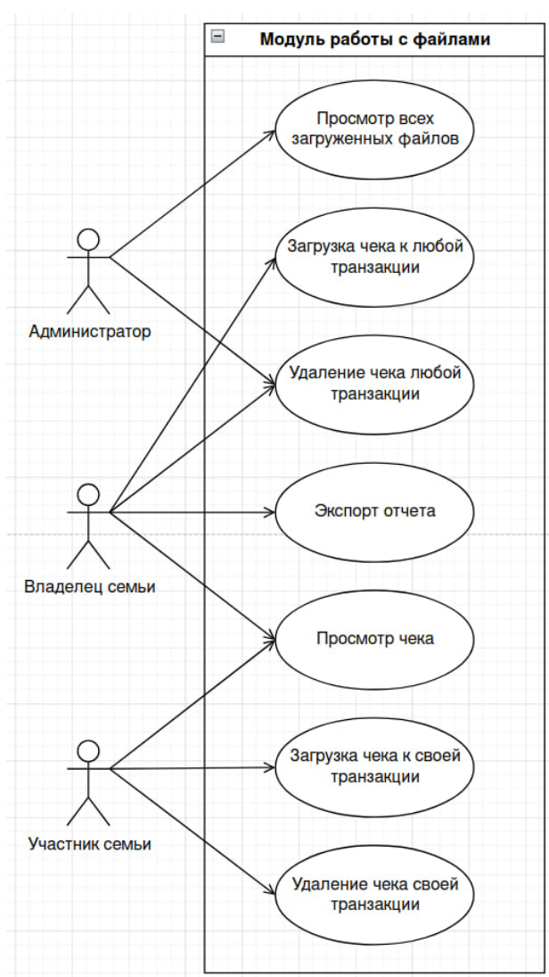
Рисунок 2.4 – Диаграмма вариантов использования модуля работы с файлами
