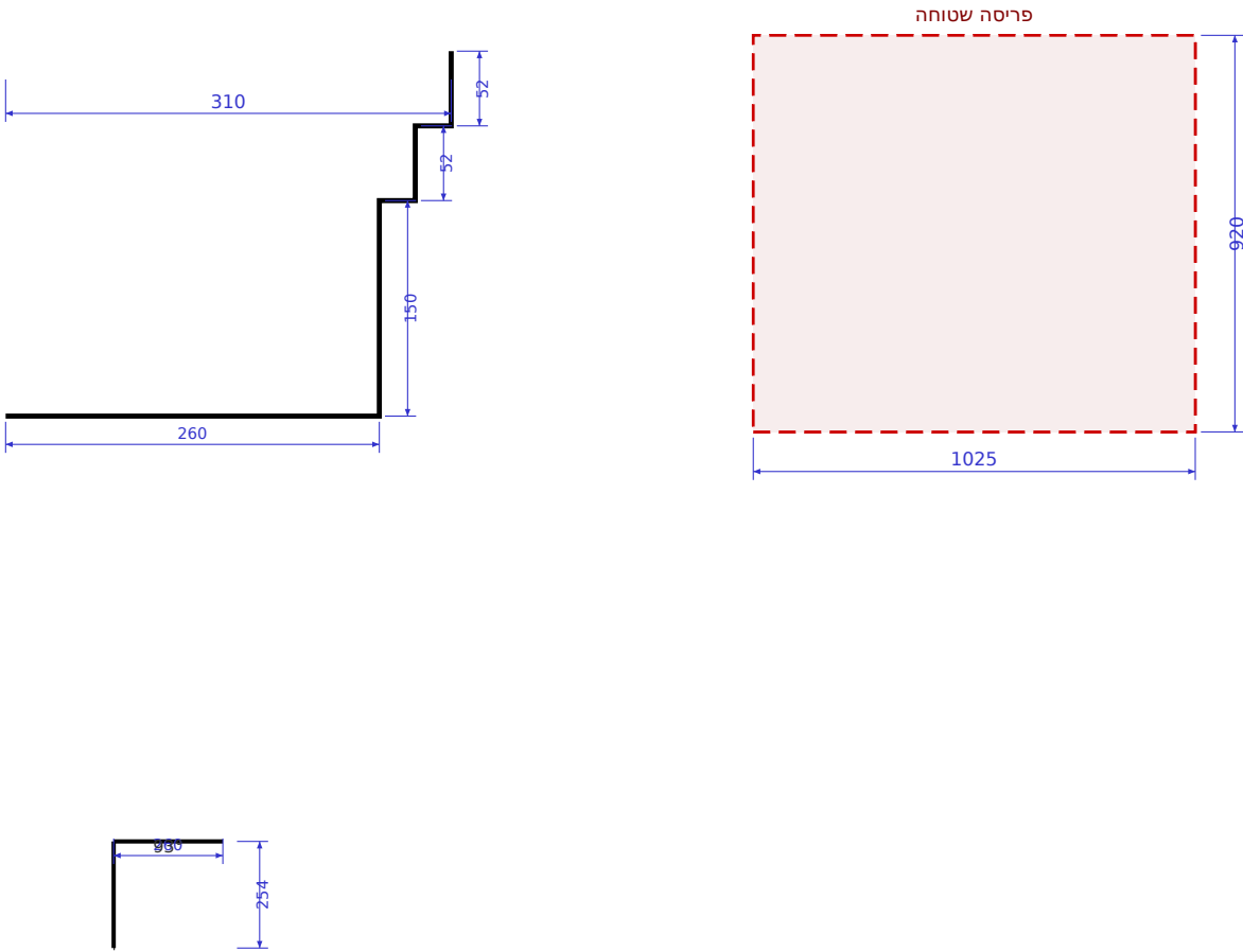
חתך פרופיל מבט צד (כפוף)
