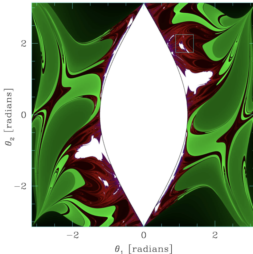
Figur 5.1: Fraktal över vilka begynnelsevinklar som gör att en dubbel-pendel vänder över, och därmed blir kaotisk. Färgkodningen i grafen visar hur fort dubbelpendeln vänder över i tidsenheter av \sqrt{l/g} . Grön motsvarar att pendeln vänder inom 10 tidsenheter, röd motsvarar 10 till 100 tidsenheter, lila motsvarar 100 till 1000 tidsenheter och blå motsvarar 1000 till 10000 tidsenheter. För mer info och bildkälla, se [12].
