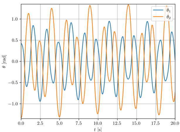
(d) Startvinklar: \theta_1 = 0.42 och \theta_2 = -1.337 [rad]. Simuleringstid: 20s.
