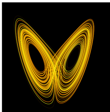
Figur 1.1: Exempel på en Lorenz-attraktor. Notera utseendet av en fjäril. Bildkälla: Lorenz system simulation . Bild av Wikimol, 2005, Wikimedia Commons. FRÅGA TILL ERIK: Hur ska man göra med källhänvisningar till bilder? Är det bättre att källhänvisa som vanligt med BibTeX(alltså att man får en siffra, precis som jag gjort med resterande källor), eller är det bättre att bara skriva källhanteringen här i bildtexten?
