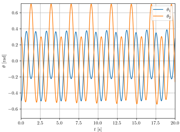
(f) Startvinklar: \theta_1 = -0.5 och \theta_2 = 0.3 [rad]. Simule- ringtid: 20s.
