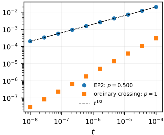
(b) Puiseux exponent
