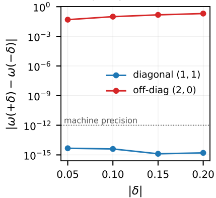
(b) \delta -parity
