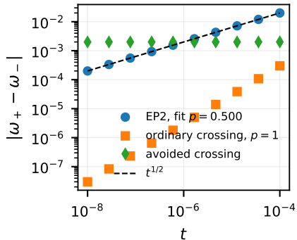
(b) Puiseux exponent
