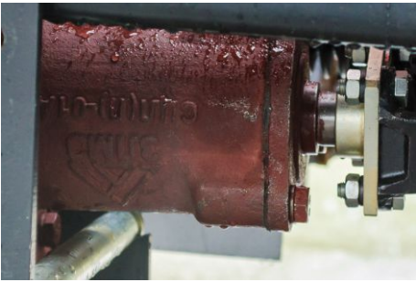
Подключение насоса через карданную передачу
