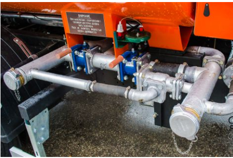
Алюминиевая сливная коммуникация
