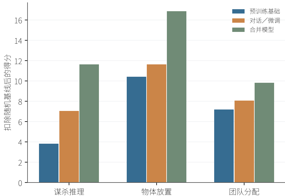
(a) 三项逐任务聚合
