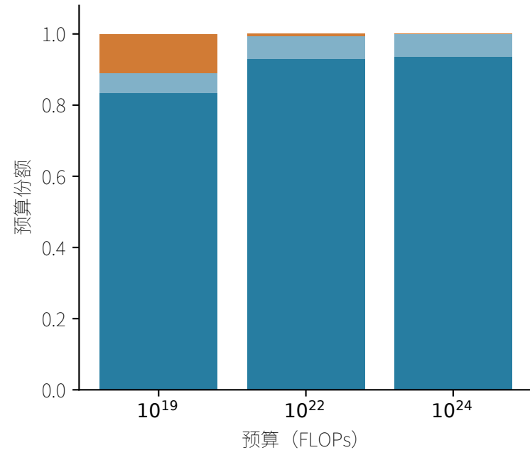
对数成本
