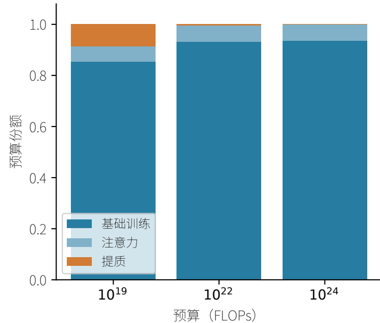
指数成本
