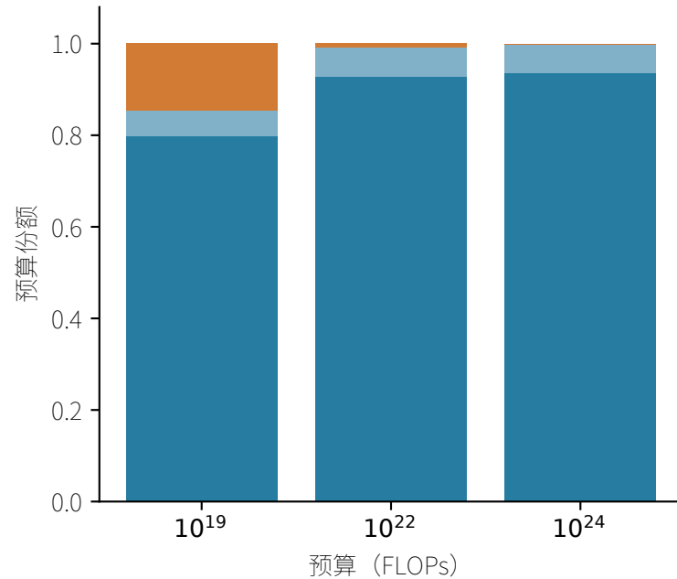
幂函数成本
