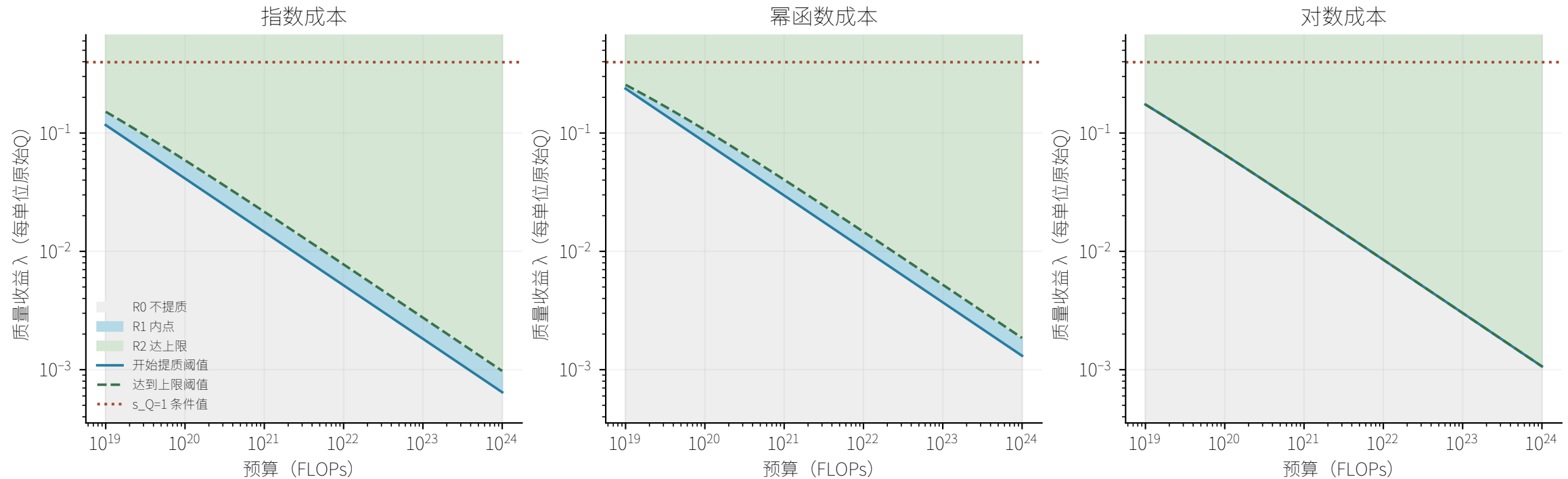
全局决策相位图 | p0, 上下文2048, 50%参照上限; 边界处允许并列最优
