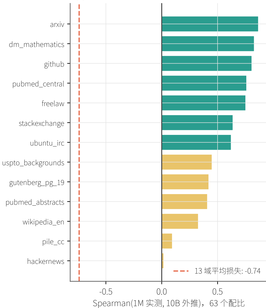
(b) 逐验证域的排序保持度：单域保持、平均反转
