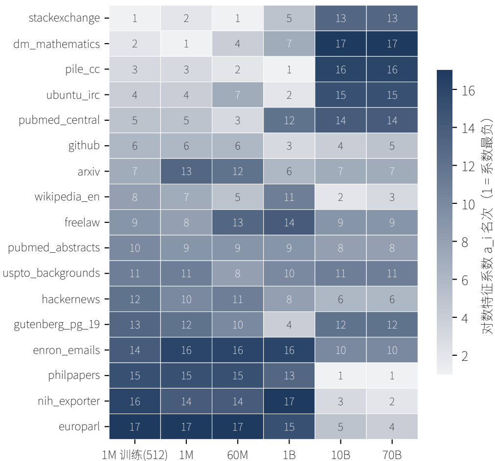
(c) 域对数特征系数名次在各尺度间的变化
