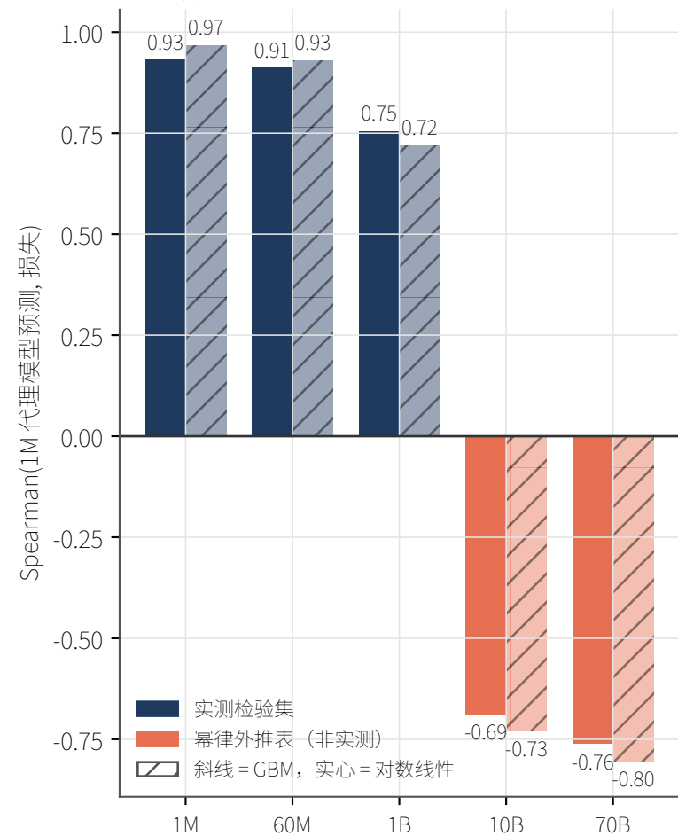
(a) 1M 代理模型的排序能力随尺度的变化
