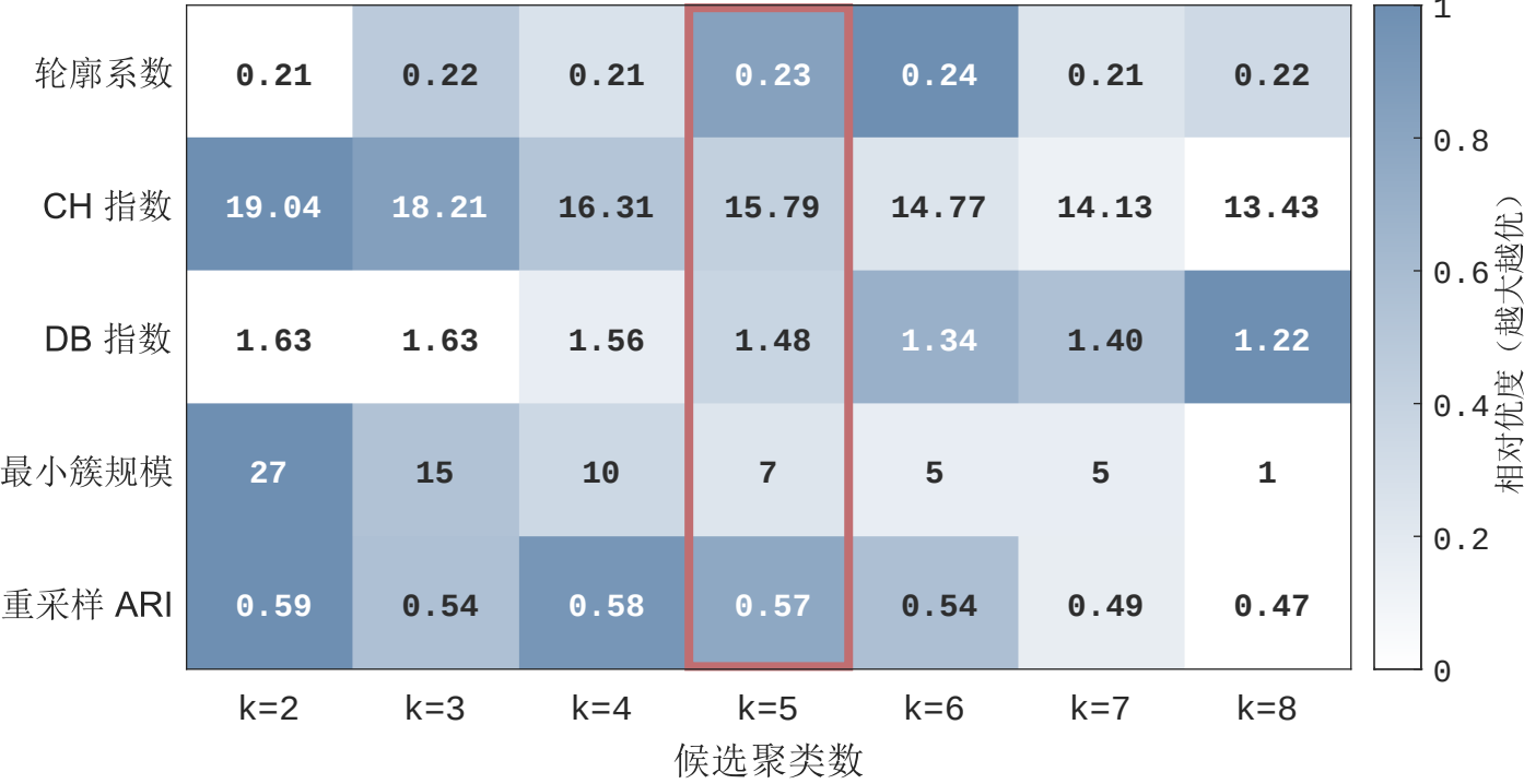
聚类数的多指标综合比较（红框为综合选择 k=5）
