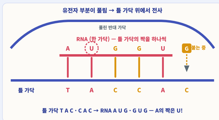
그림 3 | 전사 — 틀 가닥 TAC...에서 RNA AUG...가 태어난다. T 자리에는 U가 들어간다
